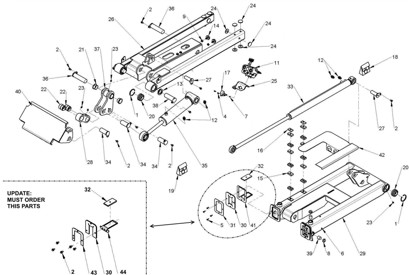
Component list [ TAV. 07 M1 SD 7-8 TELESCOPIC BOOM ]
