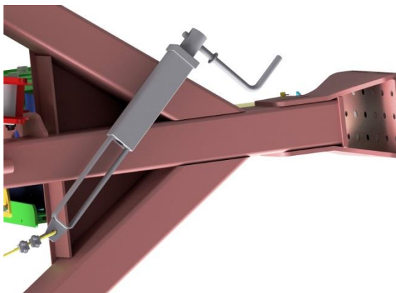
14 - Направляющая троса управления ручного тормоза
