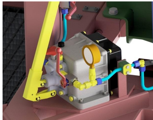
16 - Гидравлический насос
