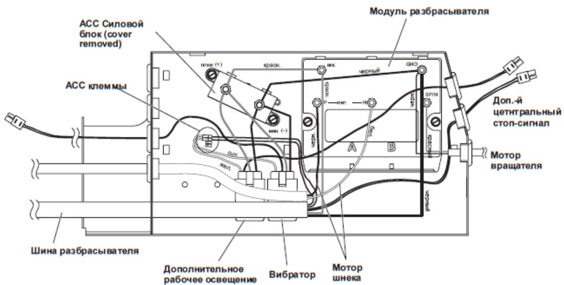
СХЕМА ЭЛЕКТРИЧЕСКОГО БЛОКА УПРАВЛЕНИЯ
