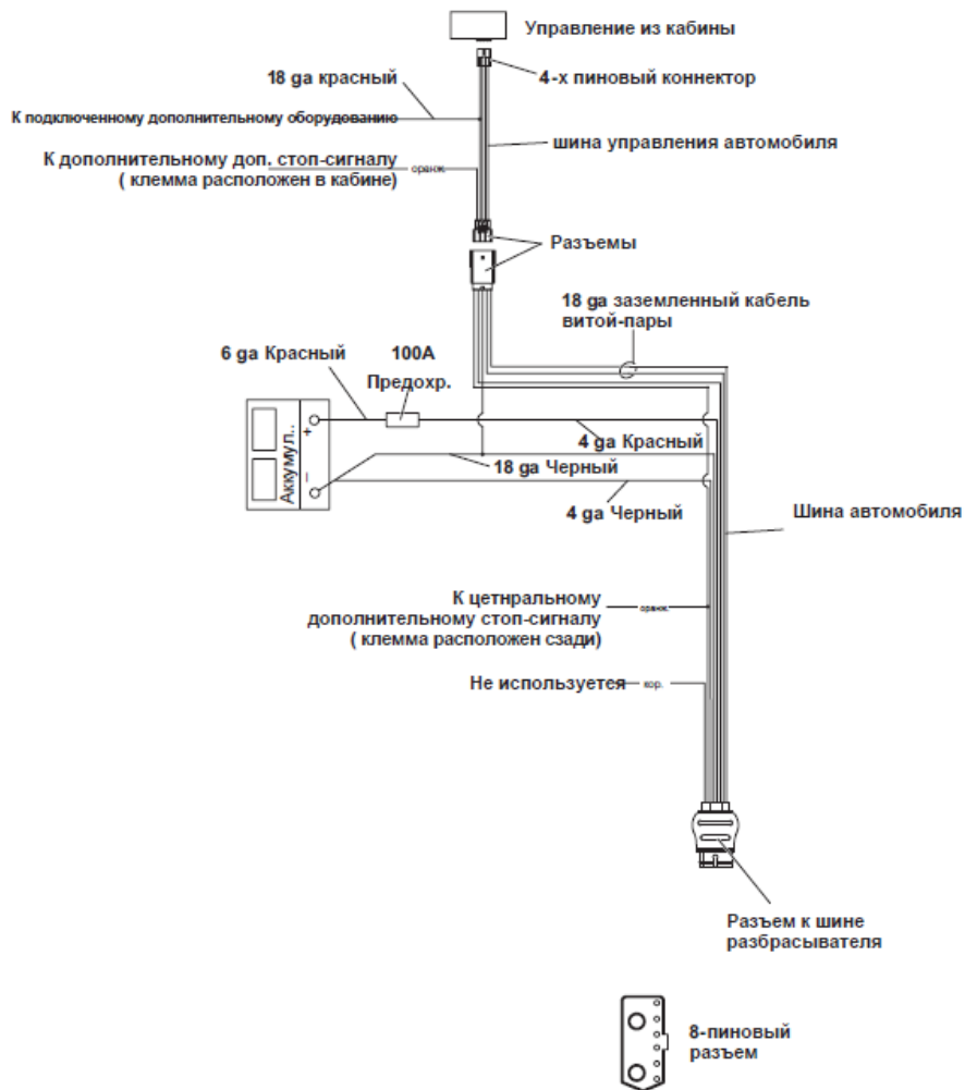
СХЕМА ПОДКЛЮЧЕНИЯ К ШИНЕ АВТОМОБИЛЯ
